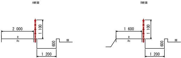
断面図 S=1:50
