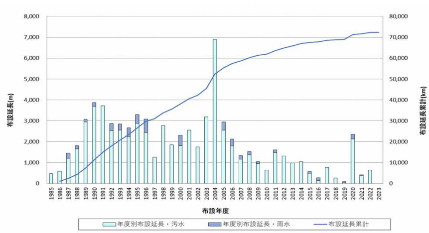
香美市の污水管ストック年度別布設延長（土佐山田）
