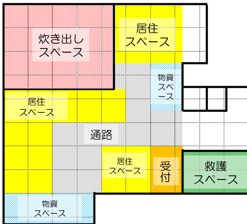
配置計画図(参考図)
