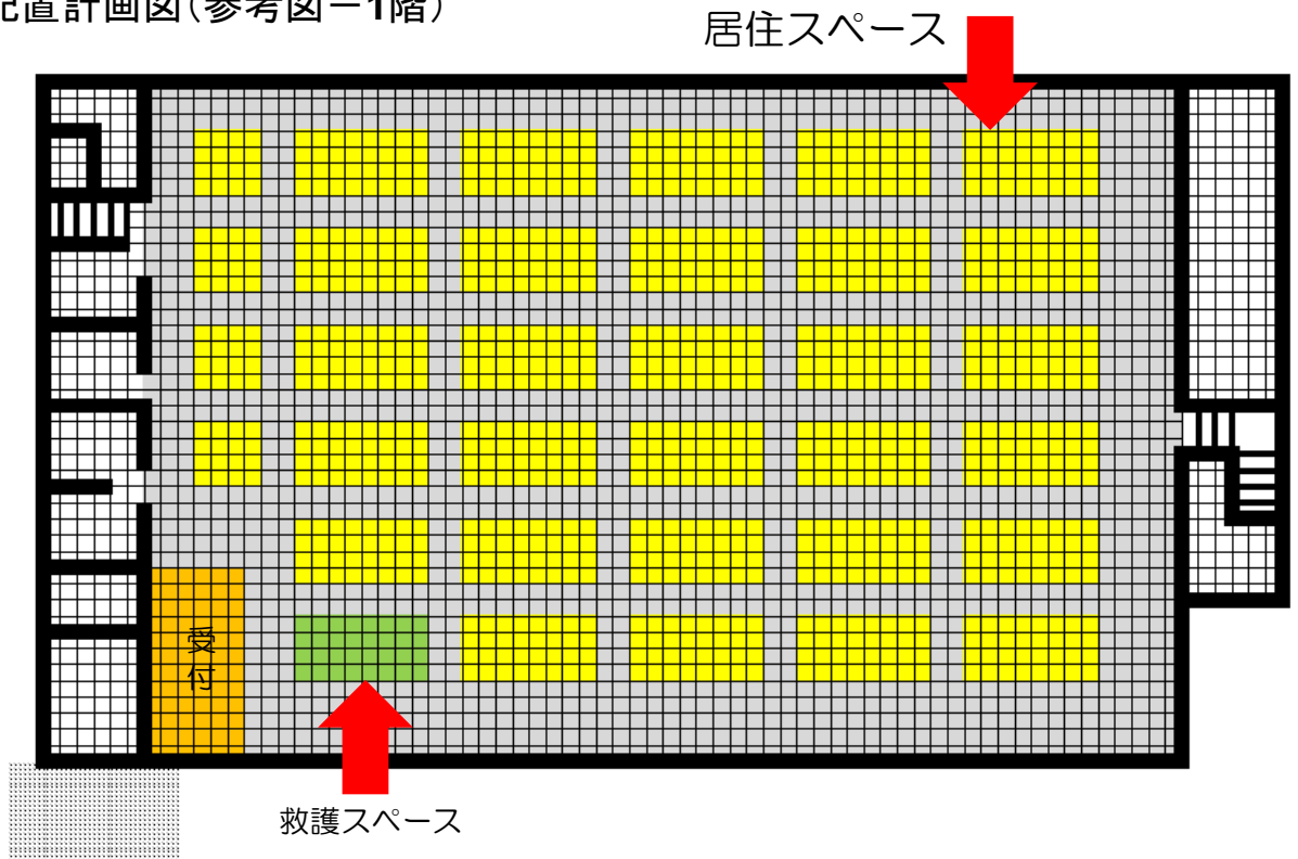
配置計画図(参考図-1階)
